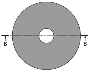
DALLE DE COUVERTURE DN 600 TROU CENTRÉ
